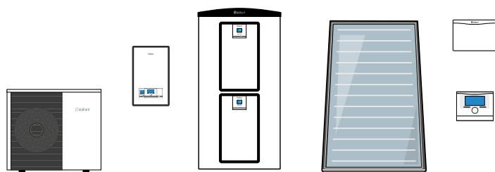
aroTHERM Split med væghængt hydraulikstation, multibeholder allSTOR eksklusiv med drikkevand og solarstation, solfanger auroTHERM plus, multiMATIC 700 og VR 920
